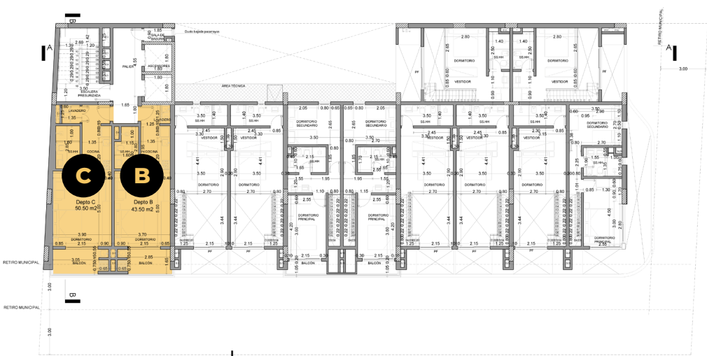
PLANTA TIPO 2 NIVEL 2 | PLANTA TIPO 4 NIVEL 4-6-8
